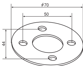
補助リング (別売)
