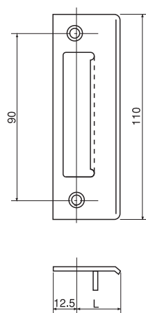
MSLストライク形状図
