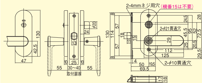
■LLK-05・15・65・68(小判座)
