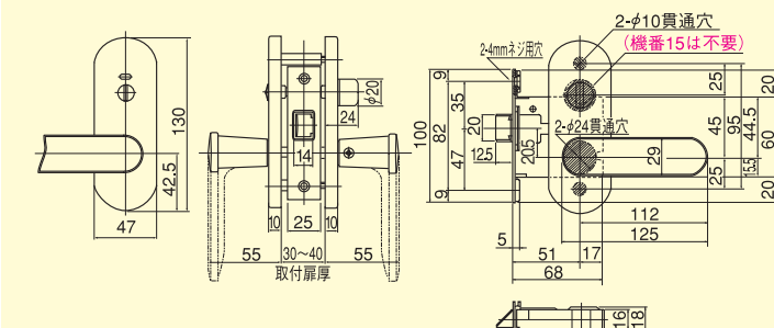
■LLT-05・15・65・68(小判座)
