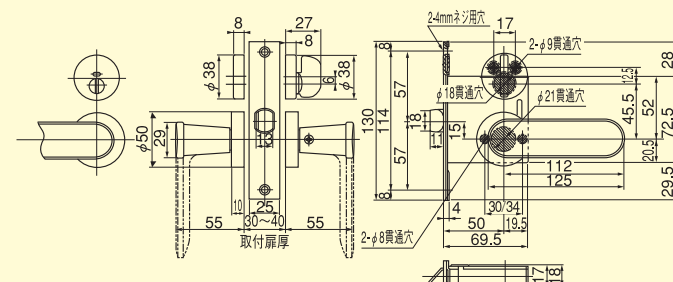
■LLK-05・65・68(丸座)
