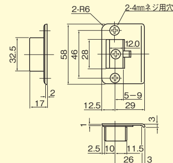
調整ストライク
