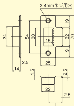
LLK・LLT用ストライク
