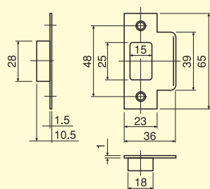
LLC用ストライク
