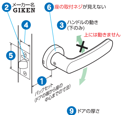
空錠(カギなし)の場合
