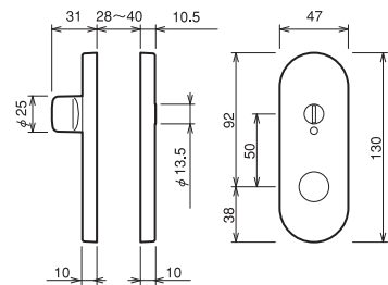
4K13小判座共通図
