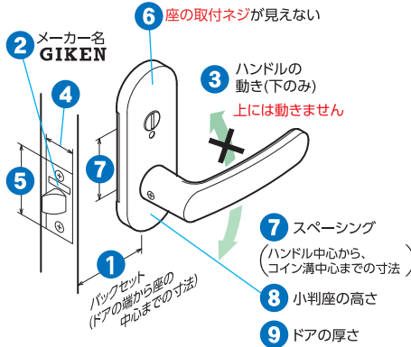
内締錠・表示錠(小判座の場合)
